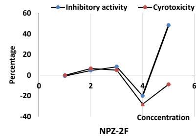
نمودار ۲: توانایی ضدویروس HIV-1 ترکیب NPZ-2F در غلظت‌های مختلف و میزان سمیت سلولی ترکیب
