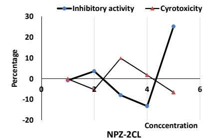
نمودار ۴: توانایی ضدویروس HIV-1 ترکیب NPZ-2CL در غلظت‌های مختلف و میزان سمیت سلولی ترکیب
